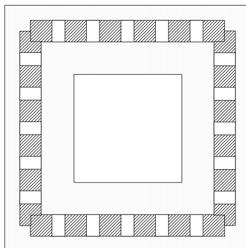
Corte em Planta
