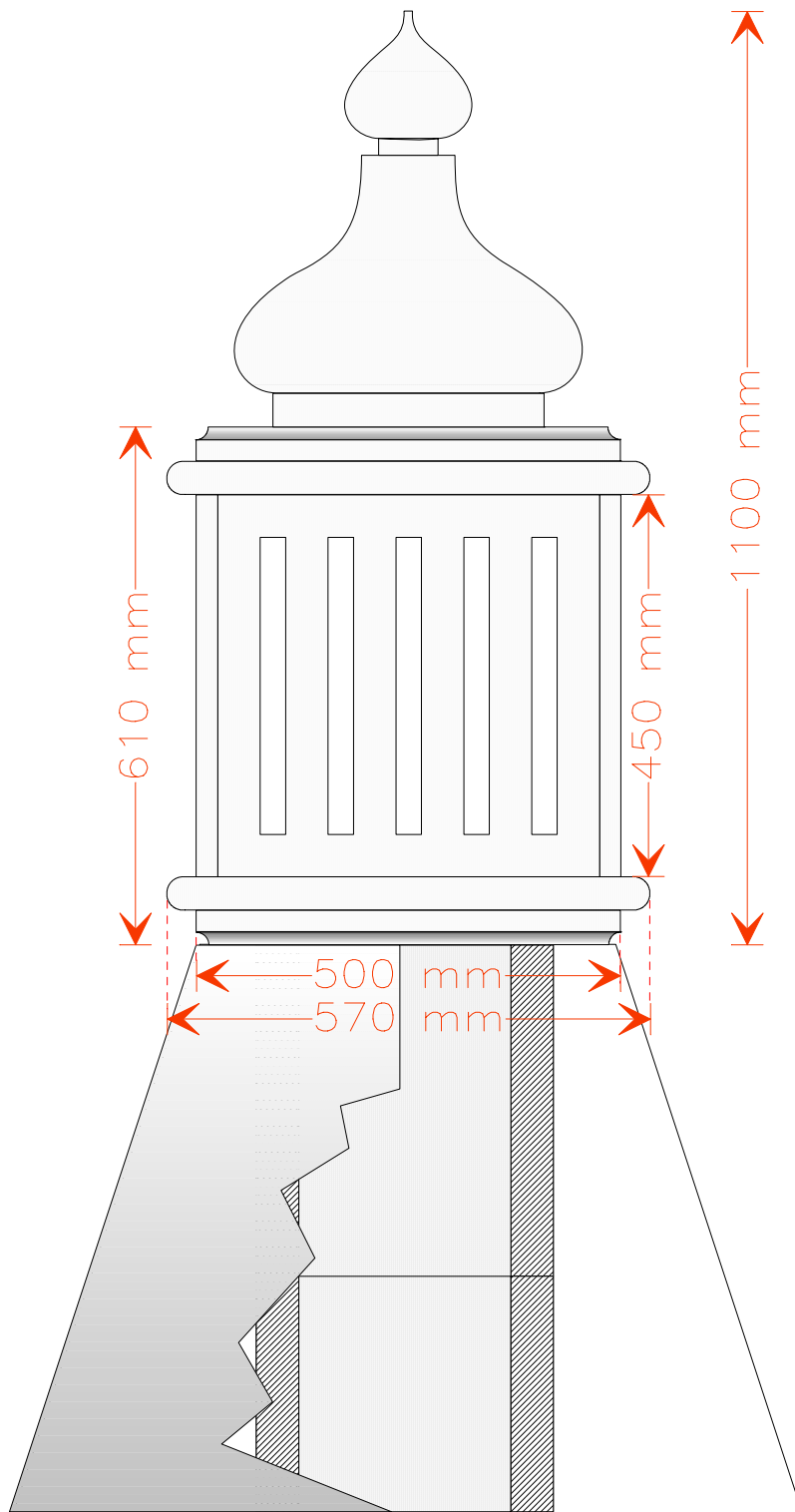
CHAMINÉ ALGARVIA NORMAL
